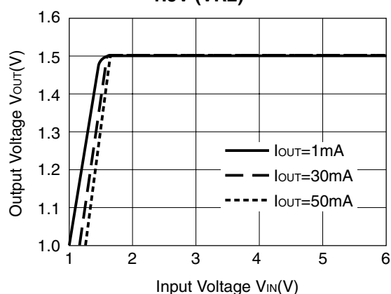
1.5V (VR2)
