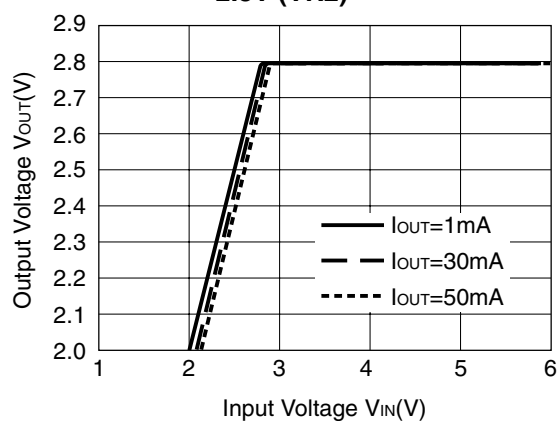
2.8V (VR2)
