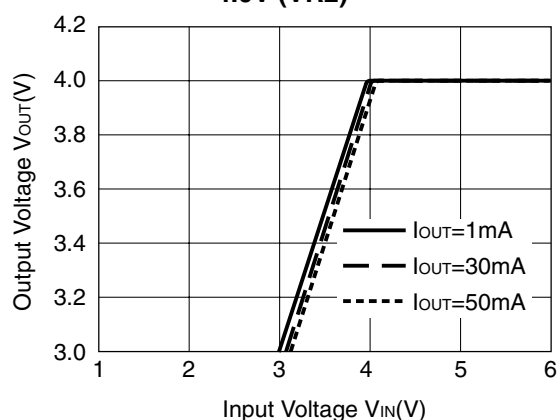
4.0V (VR2)
